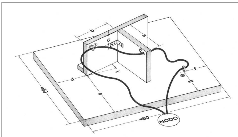
figura 1: Rappresentazione assonometrica del manufatto completo
